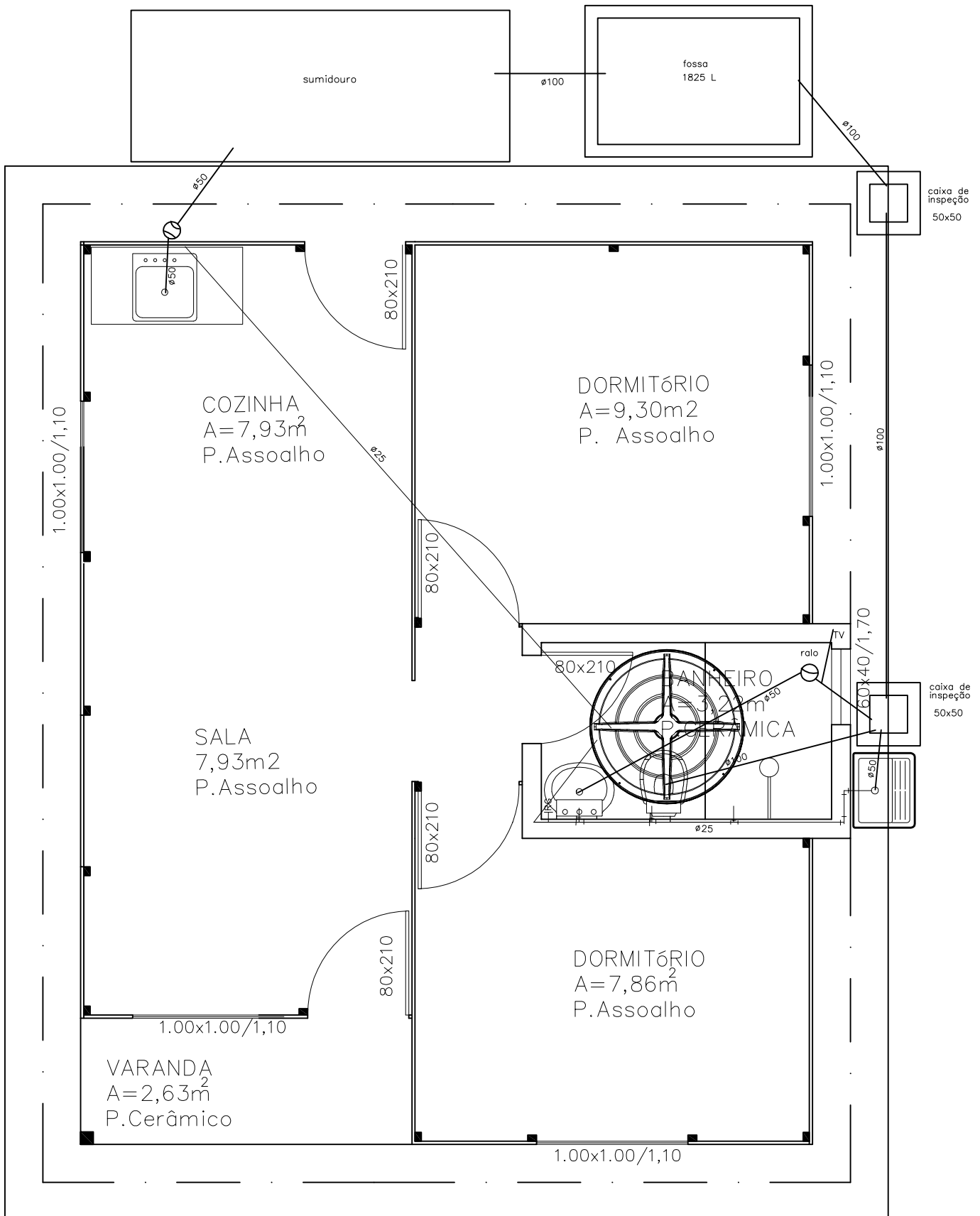
PLANTA BAIXA 41,98m 2
